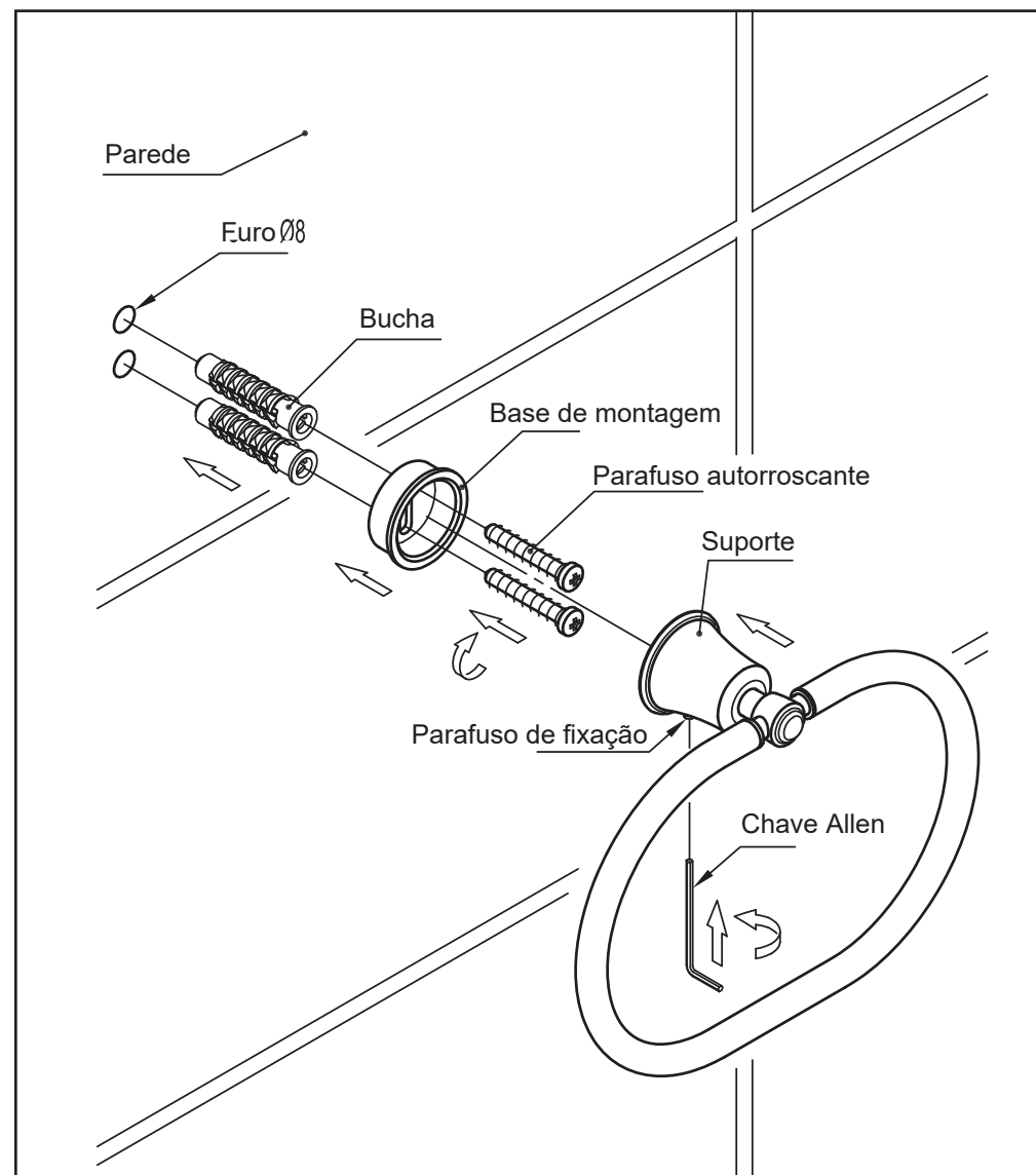
Diagrama de Instalação
