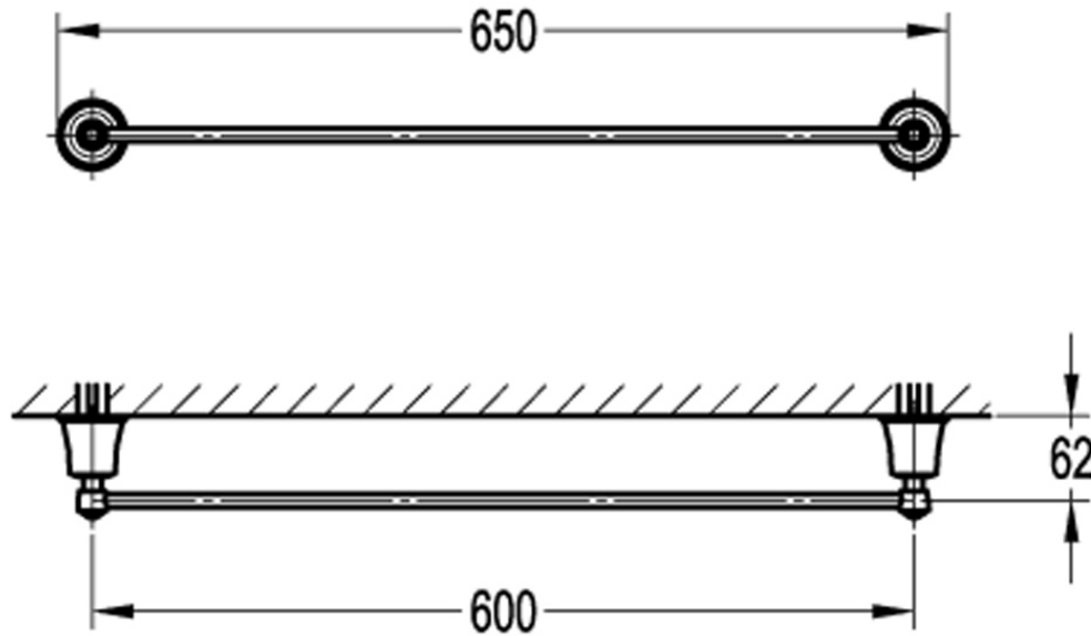
Desenho Técnico
